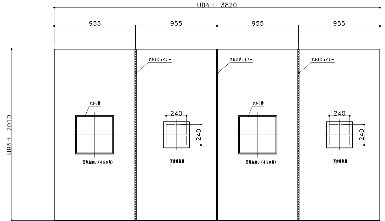
天井伏図
