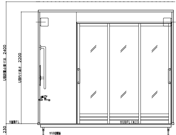
C面
