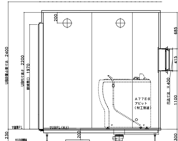
D面
