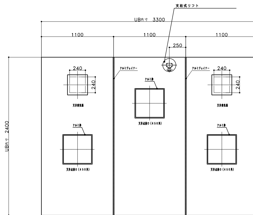
天井伏図
