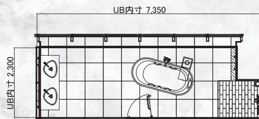
必要床下:350mm ※立上配管の場合
