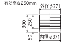
マンホールソケット (R用) H250 (有効) B33701R 5,500円
