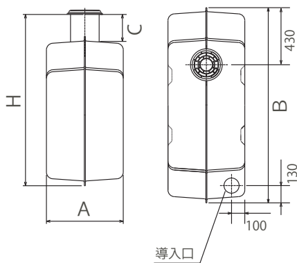
便槽寸法表
