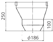
便器受け(スパット) (R用) B30301R 1,760円
