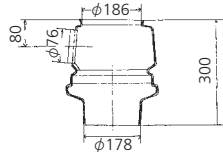
臭溜り (R用) B30401R 4,800円
