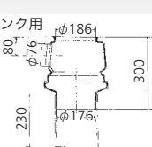
臭溜り (NP用代替品) B30401A 5,000円
