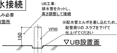
配管立ち上げ例
