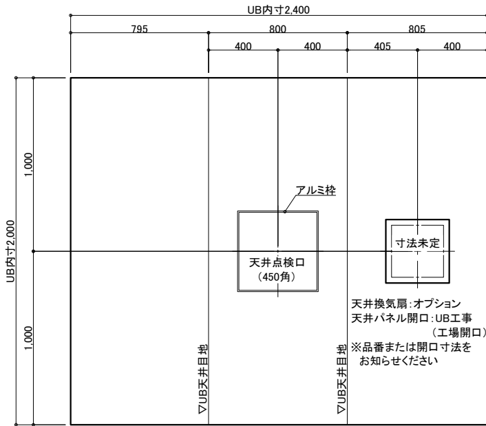
天井伏図
