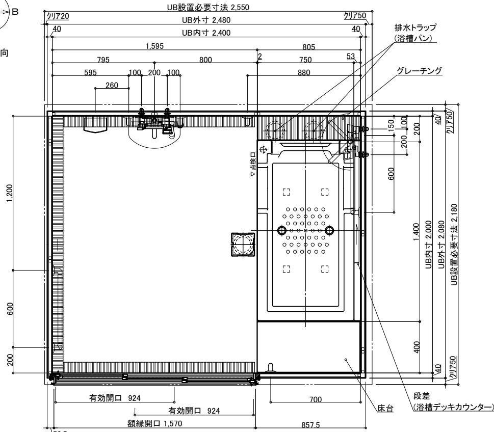
平面図
