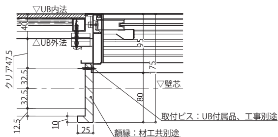
RC・S造 ■平面
