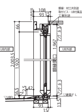
内観図 (本図はLタイプです)
