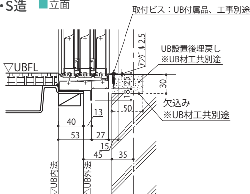
RC・S造 ■立面
