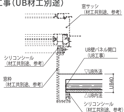
サッシ工事(UB材工別途)
