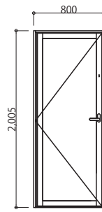
内観図 (本図はRタイプです)
