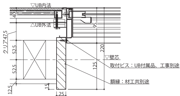
木造 ■平面
