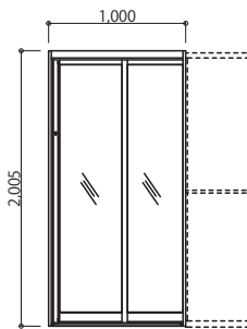
内観図
