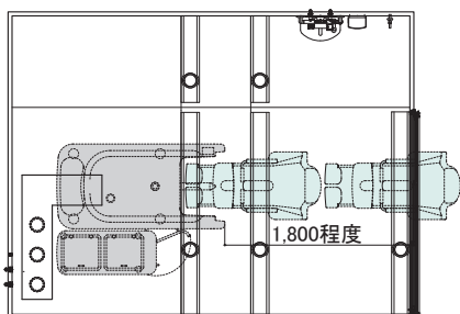
3,000mm×4,000mm (SYK3040C) 参考プラン P72
