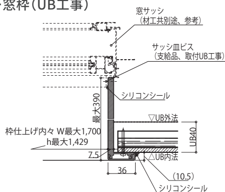
フリー窓枠(UB工事)
