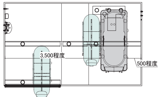
3,000mm×5,000mm (SYK3050N) 参考プラン P70
