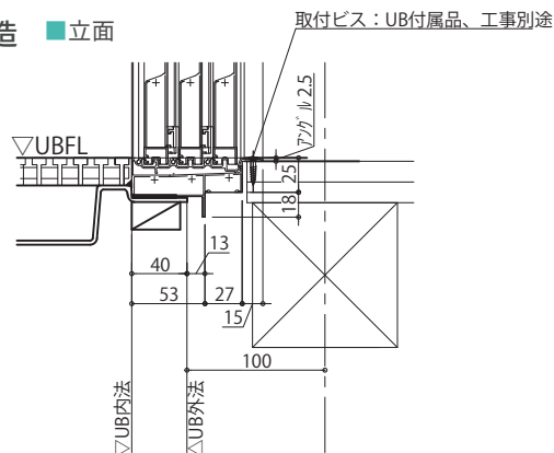
RC・S造 ■立面(置床)
