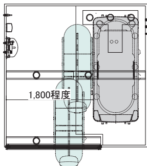
3,000mm×3,000mm (SYK3030N) 参考プラン P68
