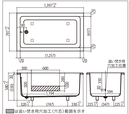
設置事例 FP-1480 (ゴム栓)
