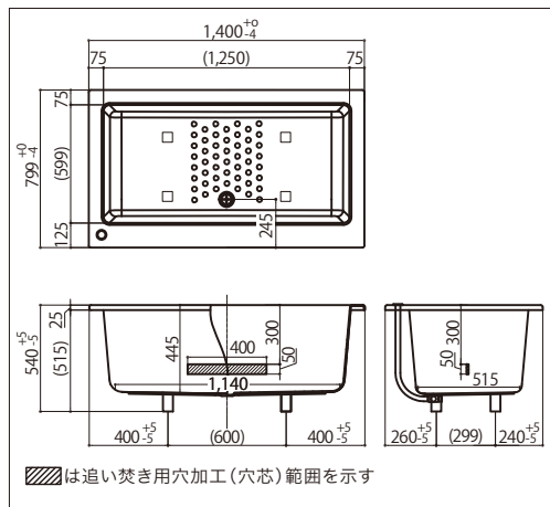
FP-1480W-WL 写真・右図面はポップアップ栓(WL) バグリップなし エプロンなし
