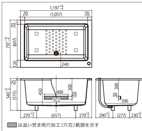
FP-1280W-WR 写真・右図面はポップアップ排水栓(WR) バグリップなし エプロンなし
