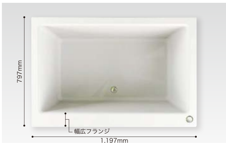
FP-1280W-WR 写真・右図面はポップアップ排水栓(WR) パーグリップなし エプロンなし
