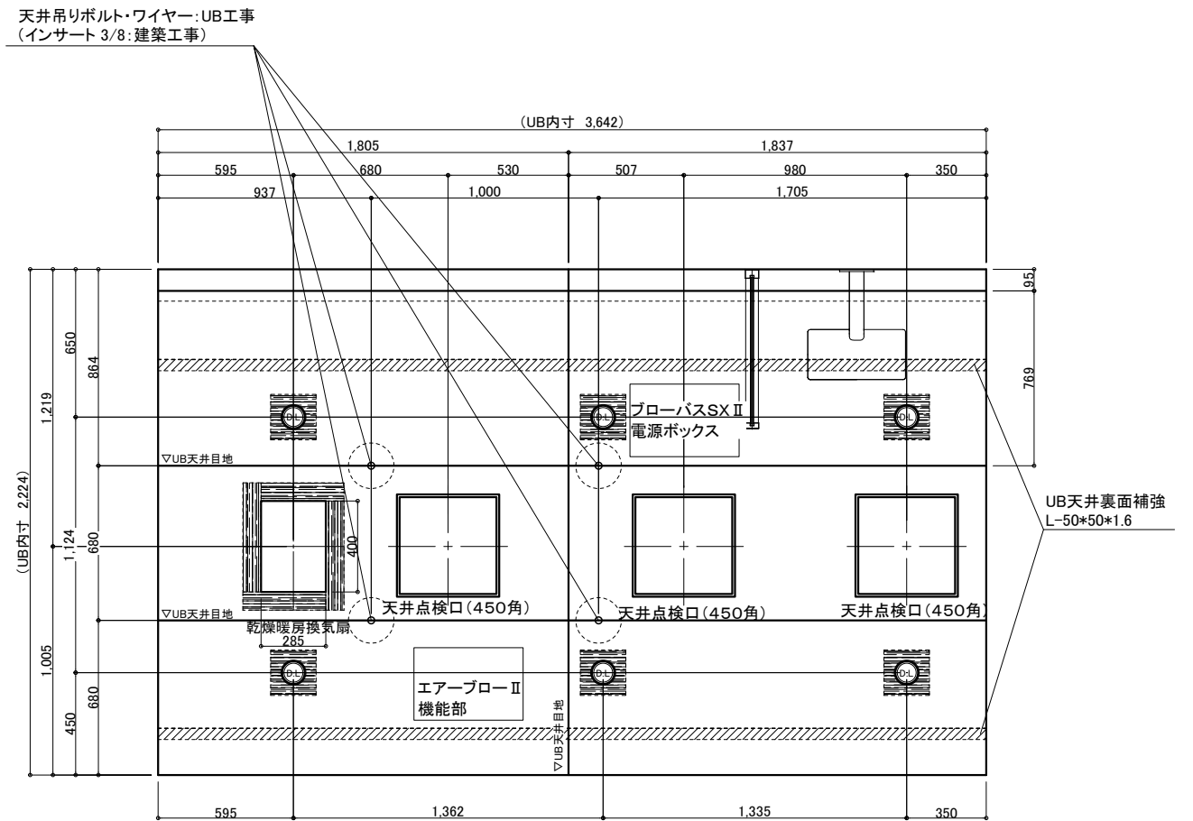
天井伏図
